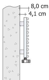
Supporto STANDARD A MURO (cod. ST)
