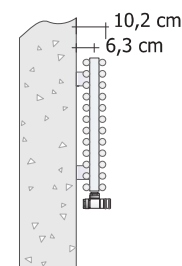
Supporto STANDARD A MURO (cod. ST)
