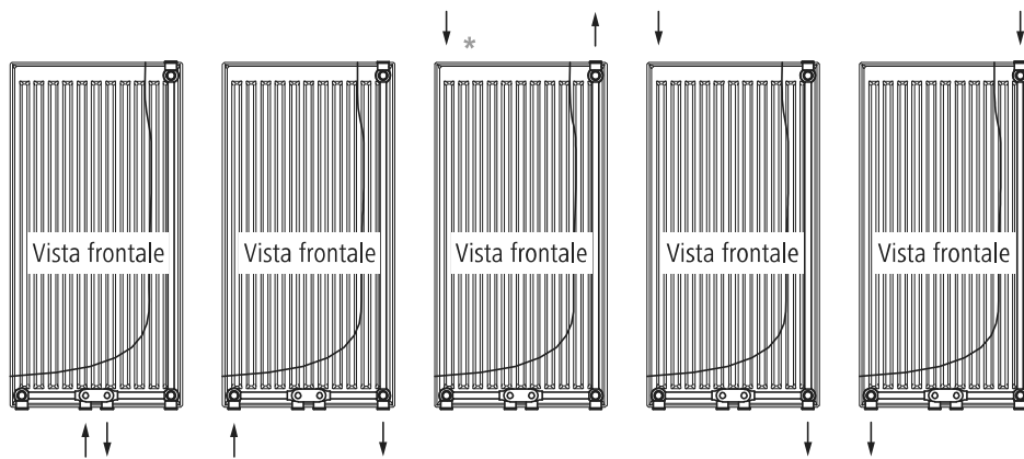
Tipo 20, 21, 22: 6 x filetti femmina G 1/2"
