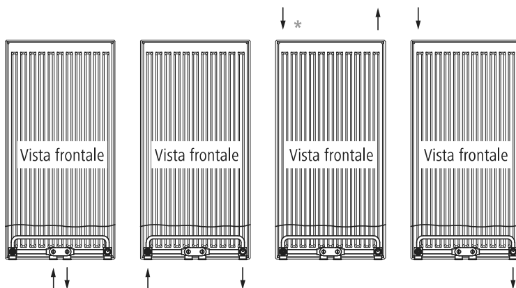
Tipo 20, 21, 22: 6 x filetti femmina G 1/2"
